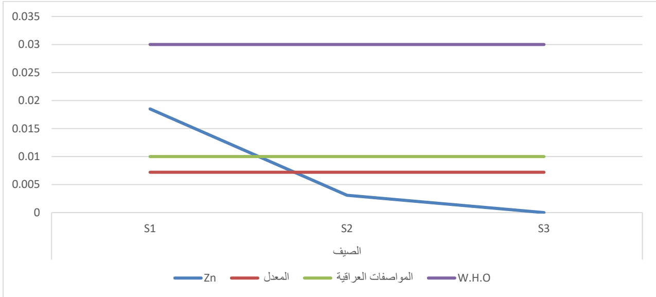
الشكل (4-30) قيم ( Zn ) والمواصفات العراقية ومواصفات منظمة الصحة العالمية ( W.H.O ) الصالحة للشرب للموسم الصيف لسنة 2023
