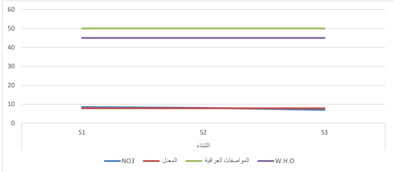
الشكل (4-28) قيم ( \text{NO}_3 ) والمواصفات العراقية ومواصفات منظمة الصحة العالمية ( \text{W.H.O} ) الصالحة للشرب للموسم الشتاء لسنة 2024
