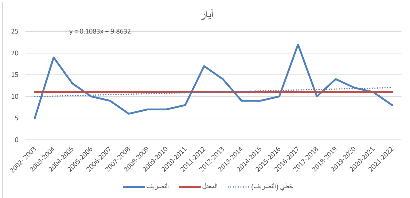
شكل (2-20) اتجاه التصاريح لشهر آيار للمدة (2002- 2022)
