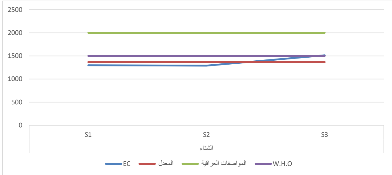
الشكل (4-12) قيم ( EC ) والمواصفات العراقية ومواصفات منظمة الصحة العالمية ( W.H.O ) الصالحة للشرب للموسم الشتاء لسنة 2024
