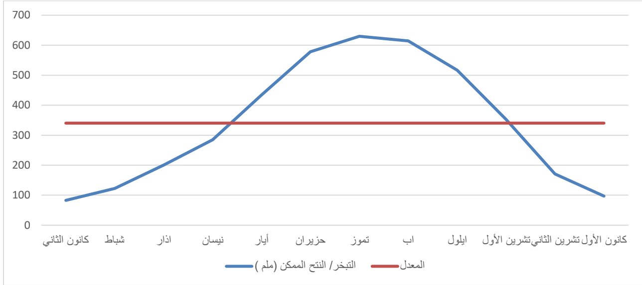
الشكل ( 1-6 ) المعدلات الشهرية لكمية التبخر/ النتج الكامن (ملم/شهر) لمحطة العمارة بحسب طريقة ايفانوف للمدة ( 1992 - 2022 )
