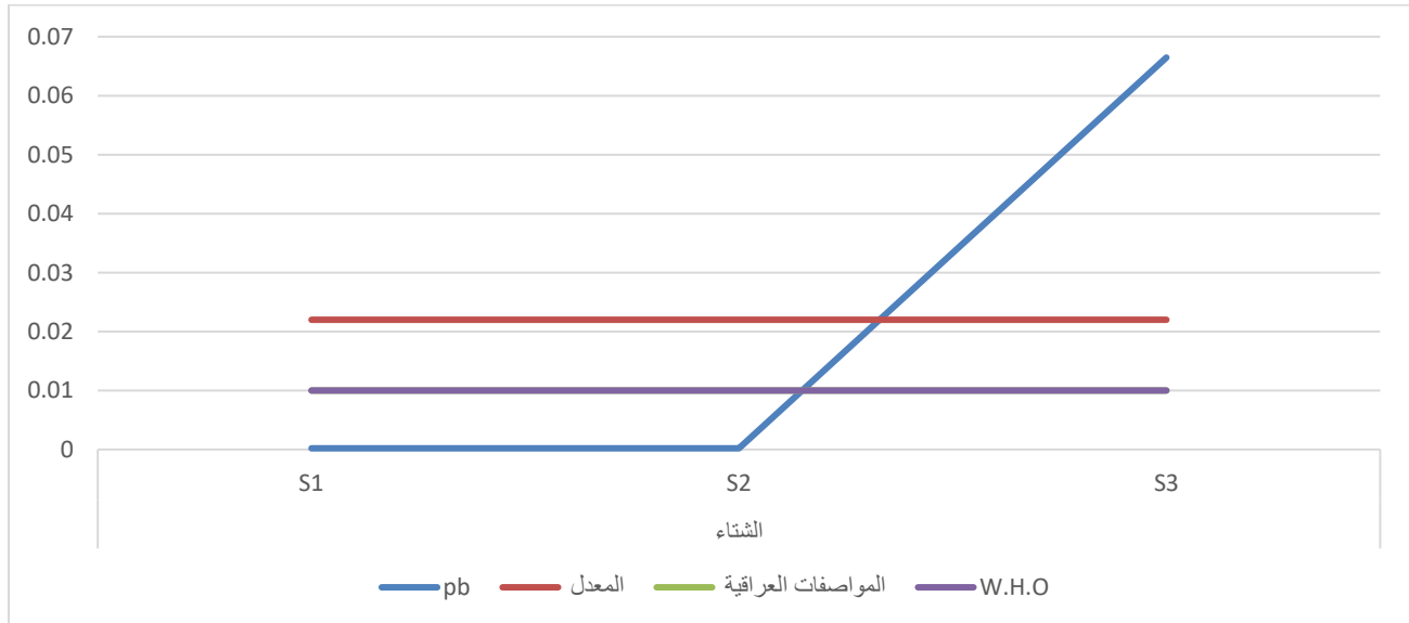
الشكل (4-33) قيم ( pb ) والمواصفات العراقية ومواصفات منظمة الصحة العالمية ( W.H.O ) الصالحة للشرب للموسم الشتاء لسنة 2024
