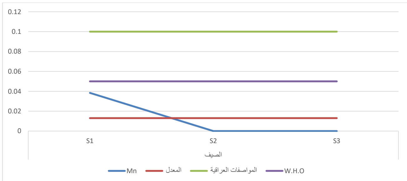
الشكل (4-29) قيم ( \text{Mn} ) والمواصفات العراقية ومواصفات منظمة الصحة العالمية ( \text{W.H.O} ) الصالحة للموسم الصيف للشرب لسنة 2023
