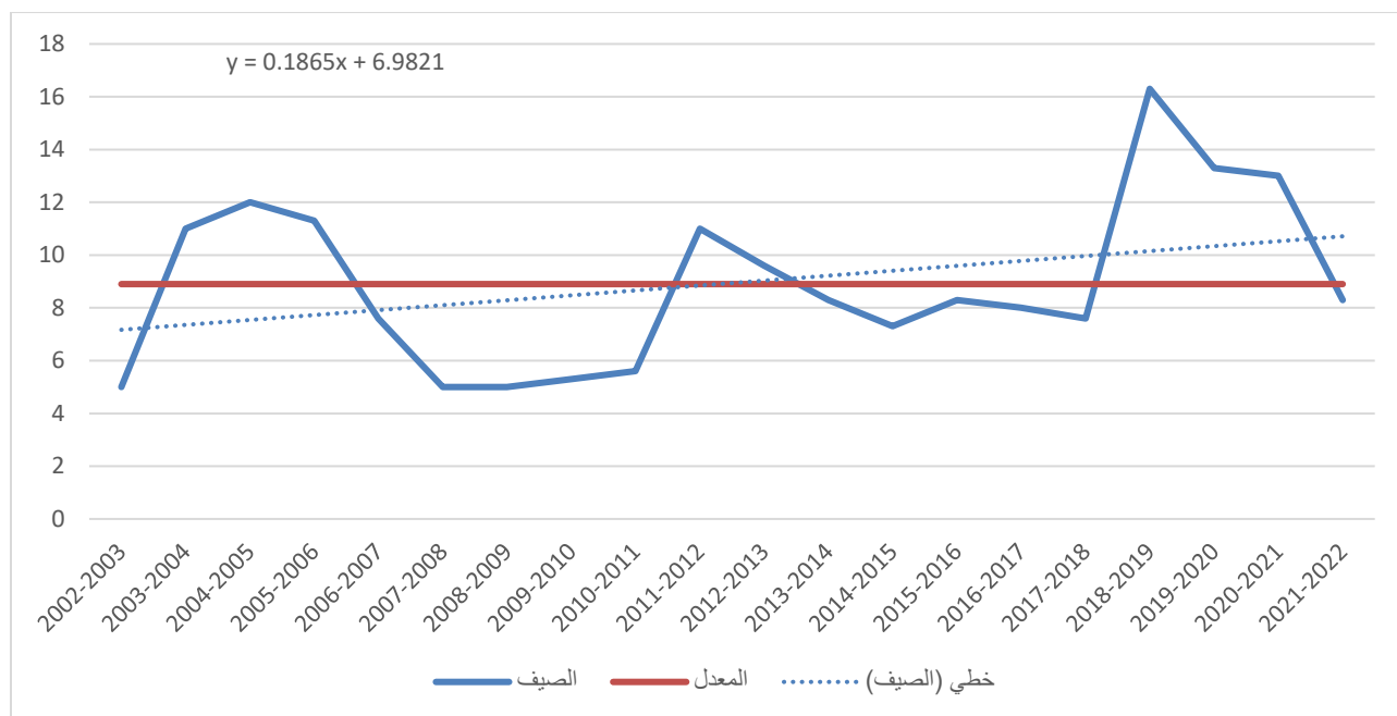
شكل (2-7) معدل تصريف فصل الصيف لنهر المشرح للمدة (2002- 2022)
