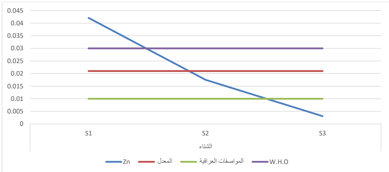
الشكل (4-31) قيم ( Zn ) والمواصفات العراقية ومواصفات منظمة الصحة العالمية ( W.H.O ) الصالحة للشرب للموسم الشتاء لسنة 2024
