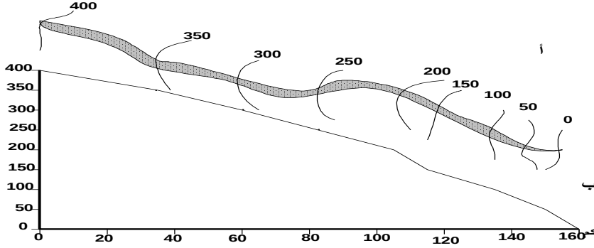
شكل رقم (5-17) مقطع طولي لمجرى نهر
