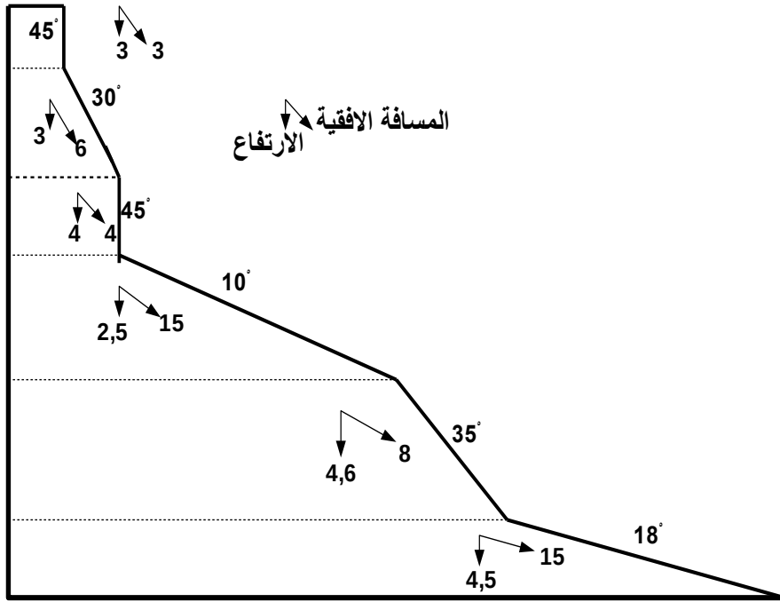
شكل رقم (3 - 43) مخطط لطبيعة منحدر
