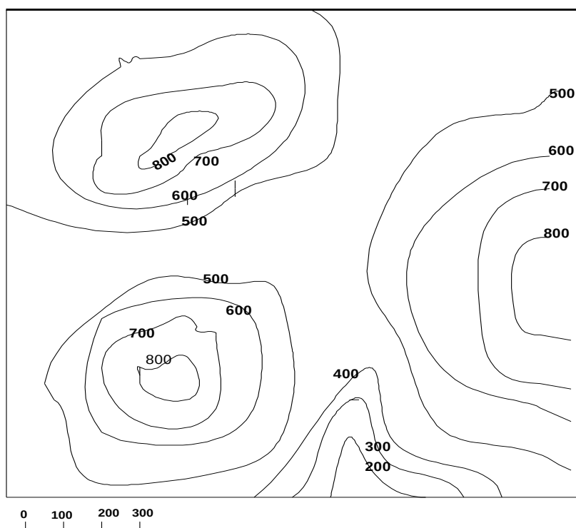
شكل رقم (2- 38 أ) - خريطة كنتورية
