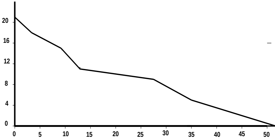
شكل رقم (3-44) مقطع طولي للمنحدر
