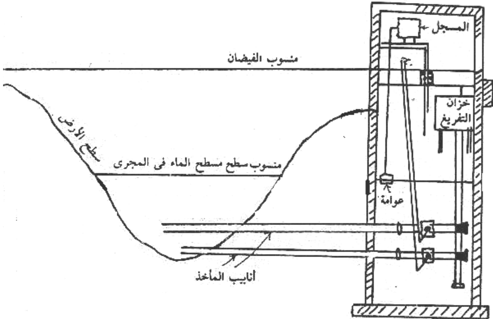
شكل رقم(26-5) مقياس مناسيب المياه الآلي
