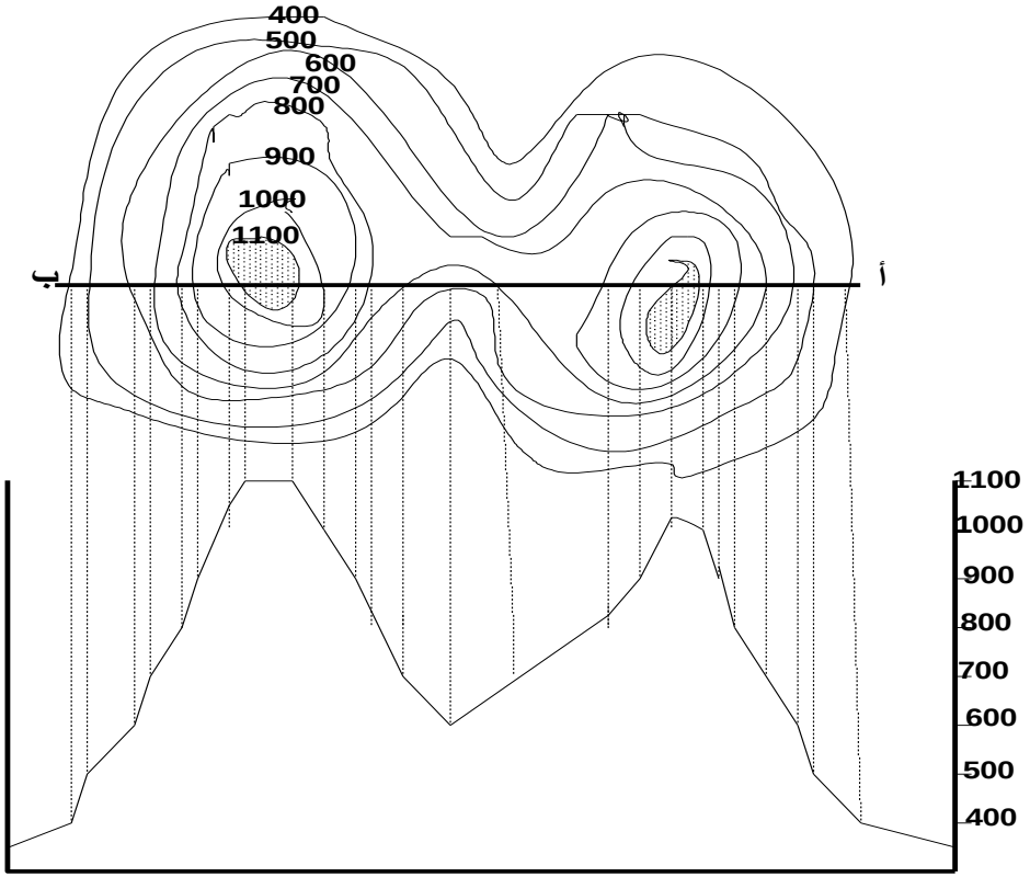
شكل رقم ( 24-1أ) مقطع تضاريسي بسيط
