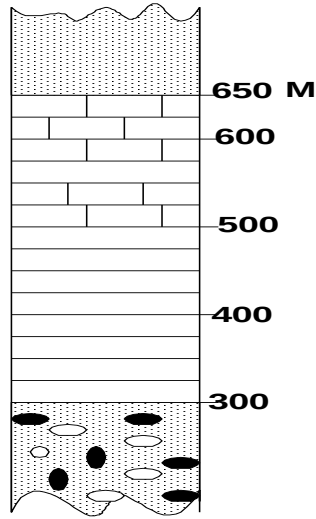
شكل رقم (38-2ج) تمثيل الطبقات الصخرية على الخريطة الكنتورية
