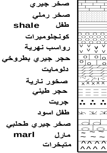
شكل رقم (35-أ) مقطع جيولوجي حسب الرموز الشائعة
