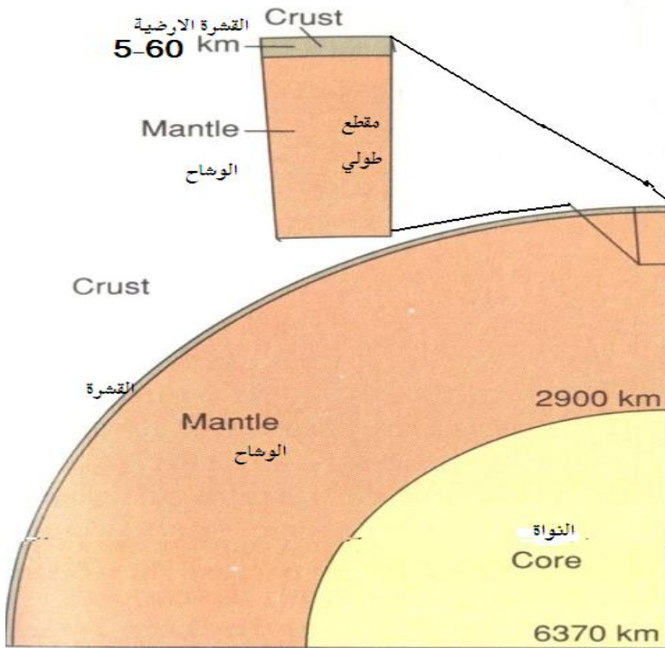
شكل رقم (4-1) مخطط لمقطع يوضح تكوينات الأرض.
