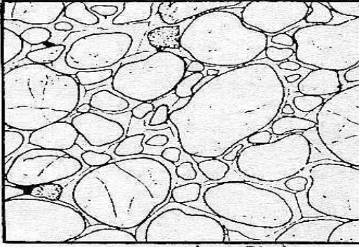
بساكنت رملی
