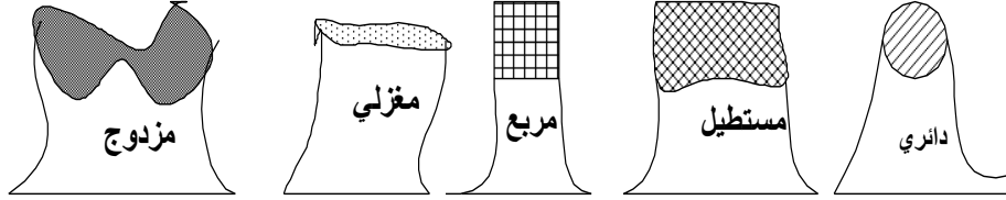
شكل رقم(3- 41) أشكال الميسات
