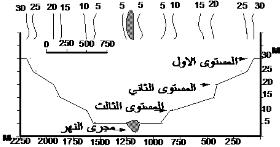
شكل رقم (5-12) يبين خطوات رسم المدرجات من الخريطة الكنتورية
