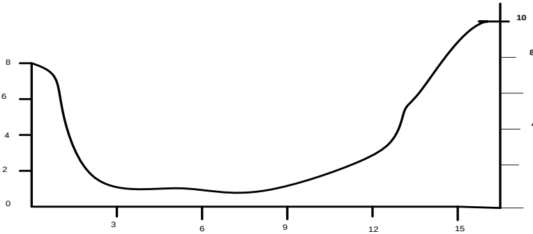
شكل رقم (5-33) مقطع عرضي لمجرى وادي
