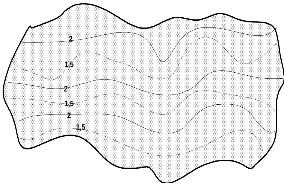
شكل رقم (7-7) توضيح خطوط التسوية الأصلية والمقترحة
