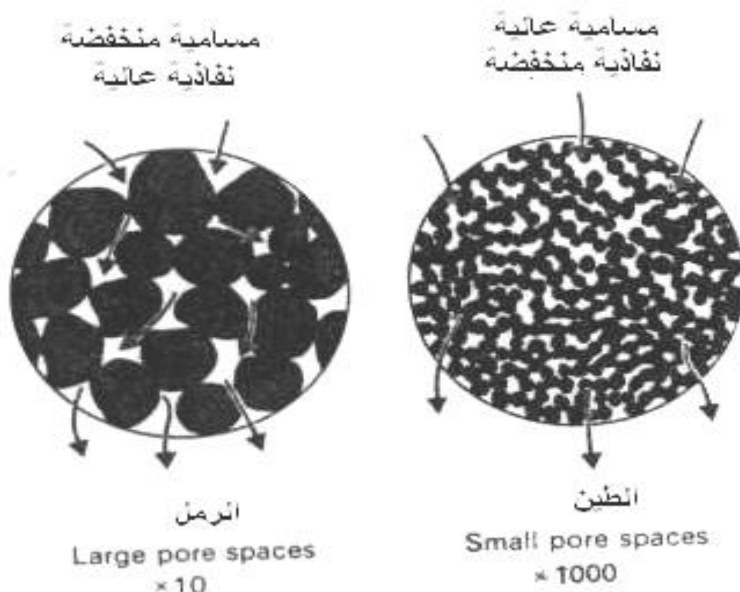
شكل رقم(2- 49) نفاذية الترب الطينية والرملية
