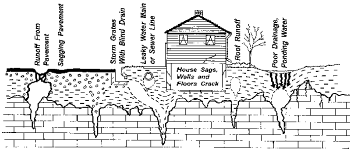
شكل رقم (23ب) هبوط مبنى
