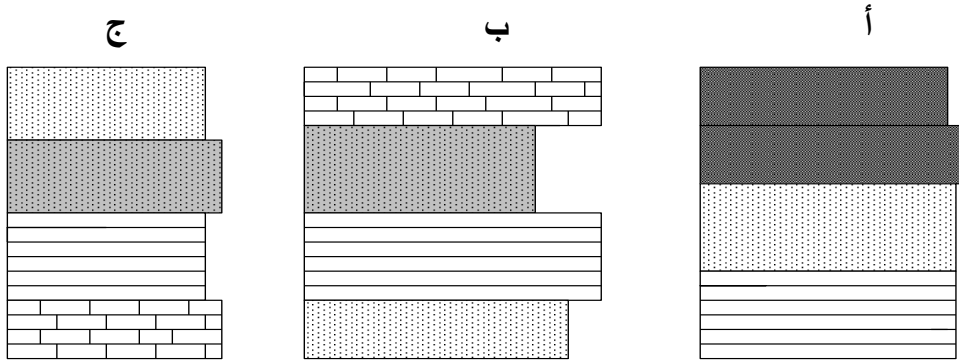
شكل رقم(34-3) امتداد الطبقات الصخرية الأفقي واثار العمليات فيها
