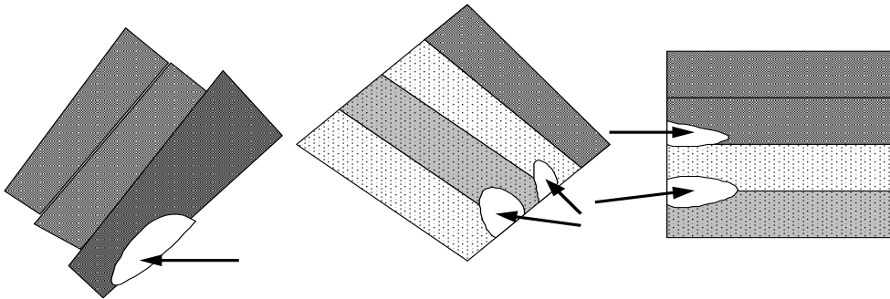
شكل رقم (4-19) أوضاع الطبقات الصخرية المكونة للسواحل
