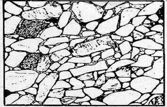
فلسبار رملی
