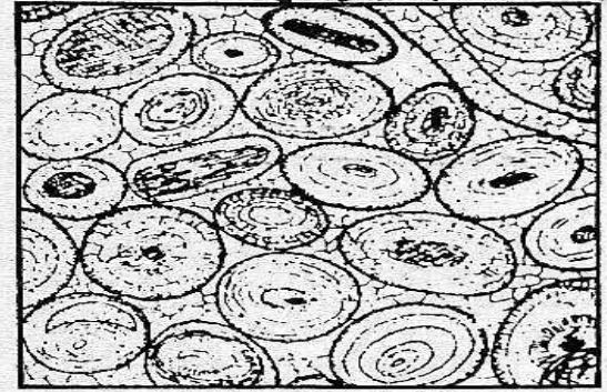
اولیت جیری
