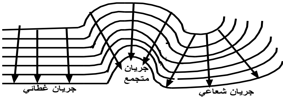
شكل رقم (4-1) العلاقة بين الانحدار والجريان
