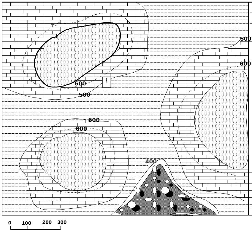
شكل رقم (38-2ج) تمثيل الطبقات الصخرية على الخريطة الكنتورية
