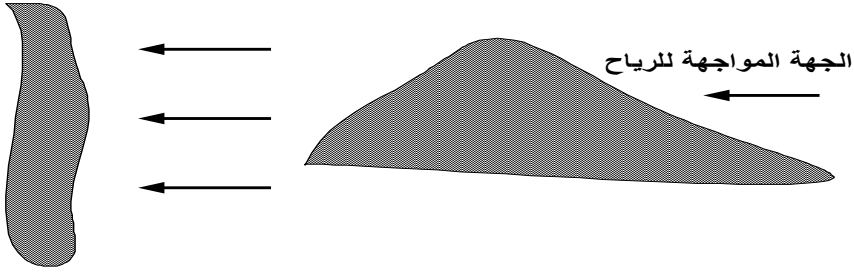
شكل رقم (3-48) تموج الكثبان الرملية
