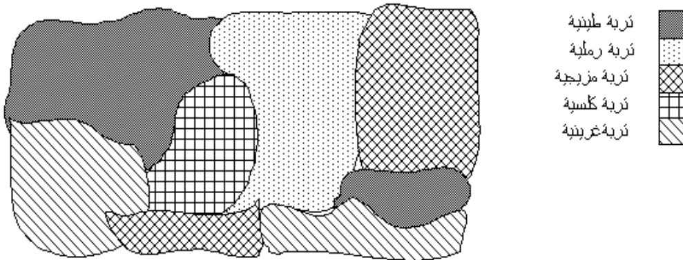
شكل رقم(2- 44) مقطع طولي يوضح أفاق التربة وسمكها
