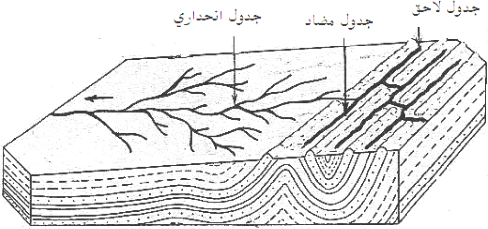
شكل رقم (5- 15) أنماط التصريف حسب ميل الطبقات
