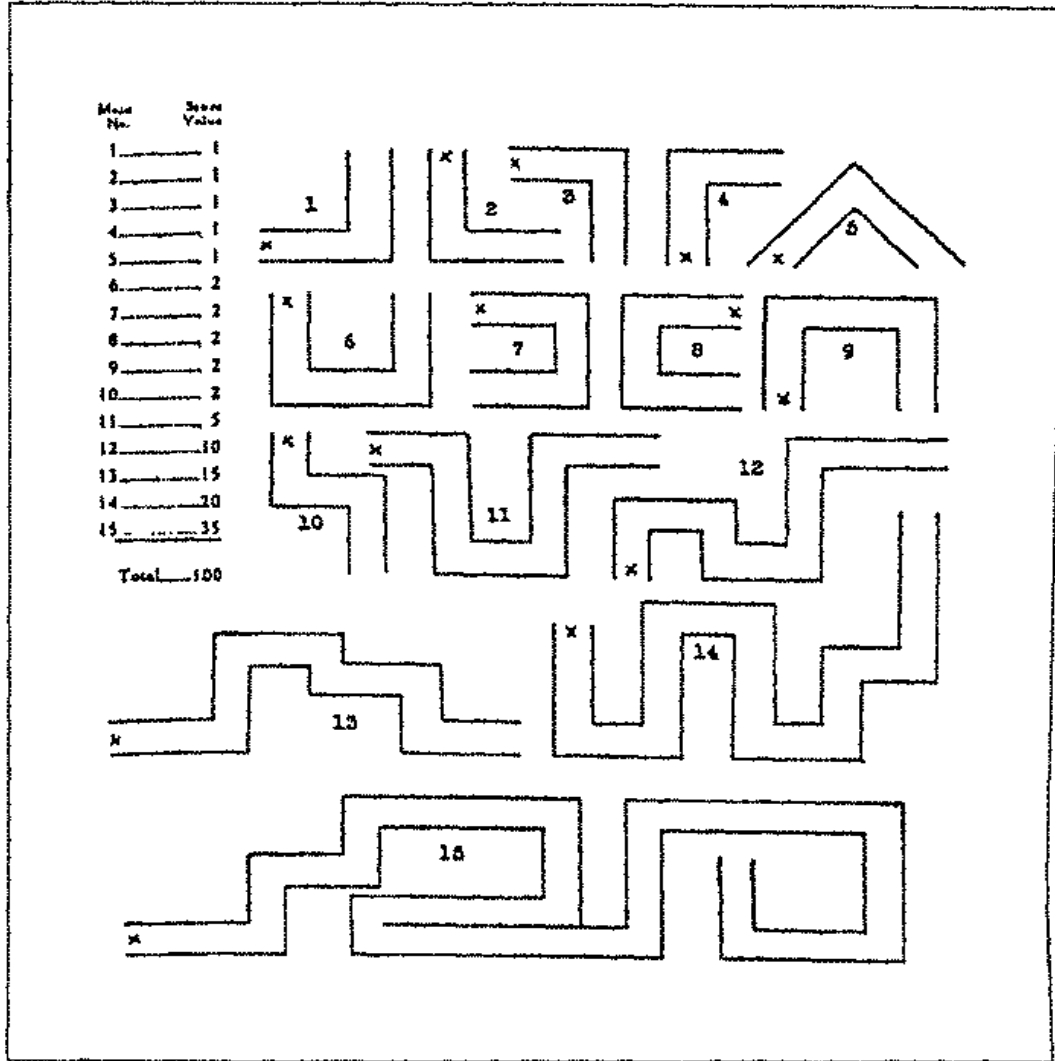
شكل (٢٠): لغز المتاهات
