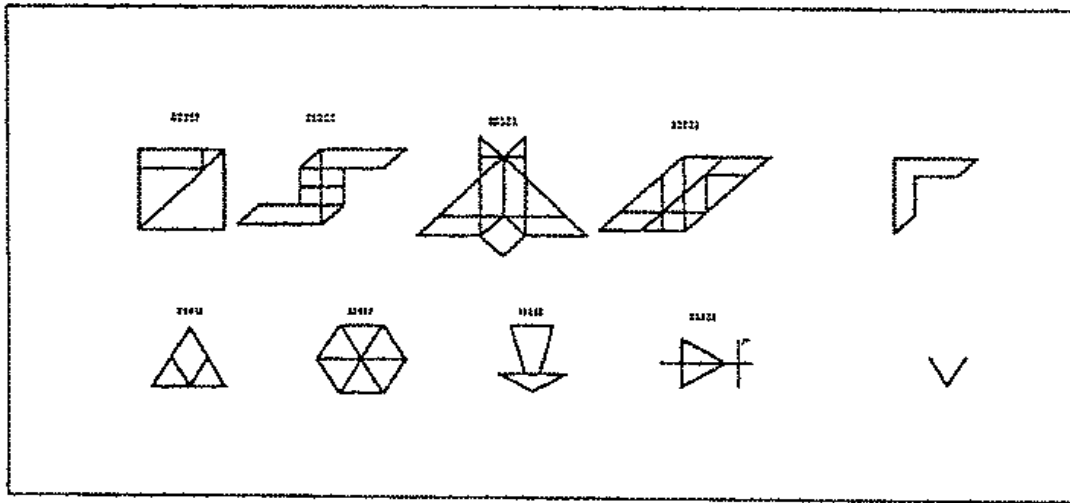
شكل (٣٠) مرونة الإغلاق : أشكال جوتشالدت : أي الرسوم الأربعة على اليمين تشتمل على الشكل الأيسر؟ (مقتبس عن : ٨ ص ٦٢٦)
