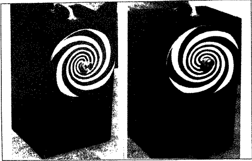
شكل (٣١) : بريمة أرشميدس :
