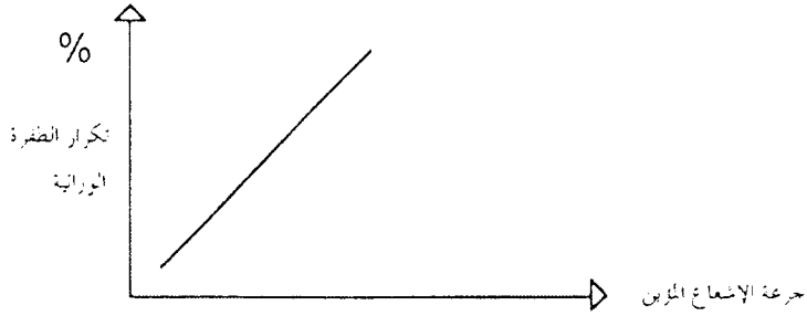
شكل ( 6 - 9 ) : العلاقة بين جرعة الإشعاع المؤين وتكرار الطفرة ويلاحظ أن العلاقة خطية بينهما حيث يزداد تكرار الطفرة بزيادة جرعة التشعيع.
