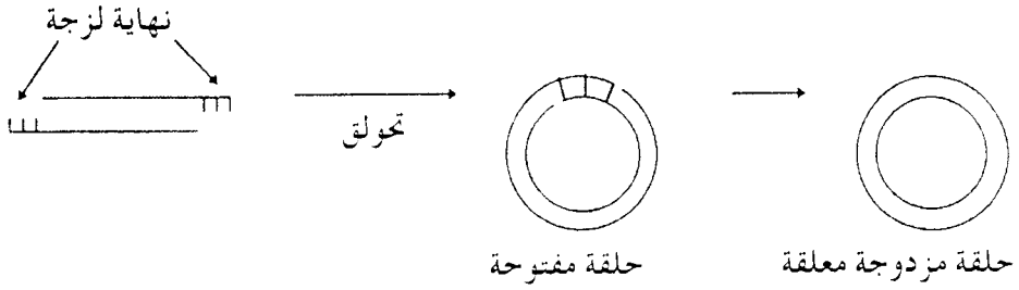
شكل (4 - 21) : DNA العائلي لامبدا الحاوي على النهايات للزرعة وآلية تحويله إلى DNA حلقي .
