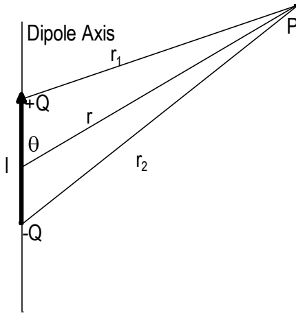
شكل (2.14) الجهد الكهربى لثنائى القطب الكهربى.
