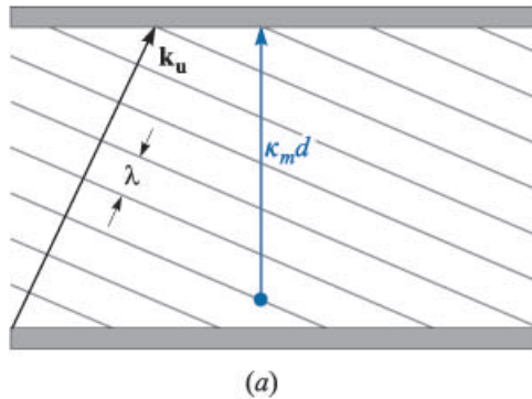
شكل (9.10) انزياح الطور للموجة الصاعدة بين لوحتي المرشد الموجي .
