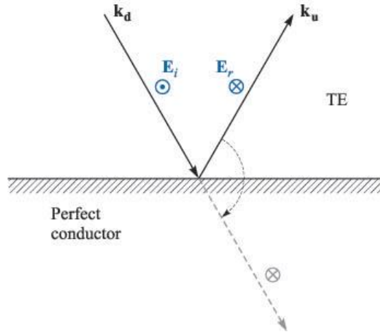
شكل(9.11) انزياح طور الموجة نمط TE عند الانعكاس عن سطح لوح تام الموصلية.
