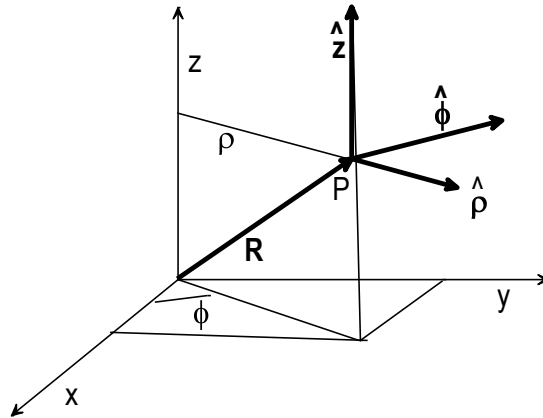
شكل (1.3) نظام الإحداثي الأسطواني.
