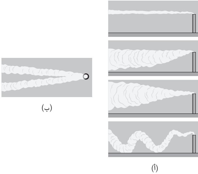
شكل ٤-١١: بند ٤-٧٥: (أ) أعمدة الدخان التي تَصْدُر من المداخل في رياح مستقرة أفقية. (ب) مسقط رأسي يبيّن عمود دخان ينقسم إلى عمودين.
