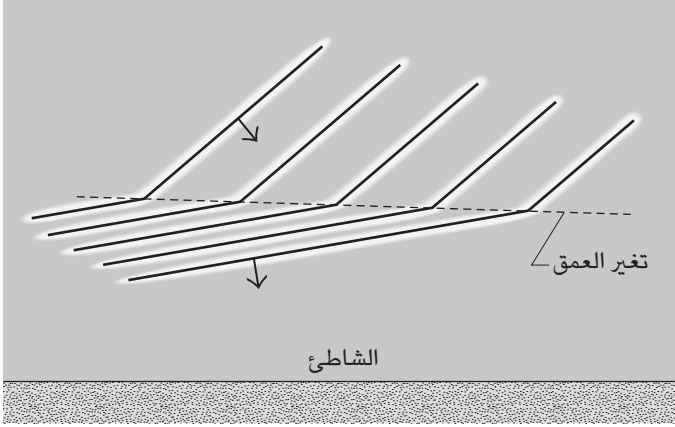
شكل ٢٠-٢: بند ٦٥-٢: منظر علوي للأمواج مُحيط تُغيّر الاتجاهات مع انخفاض عُقَم الماء.
