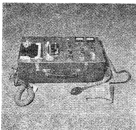
جهاز تسجيل الاستجابة الخلفية ويستخدم في تجارب الانفعالات
