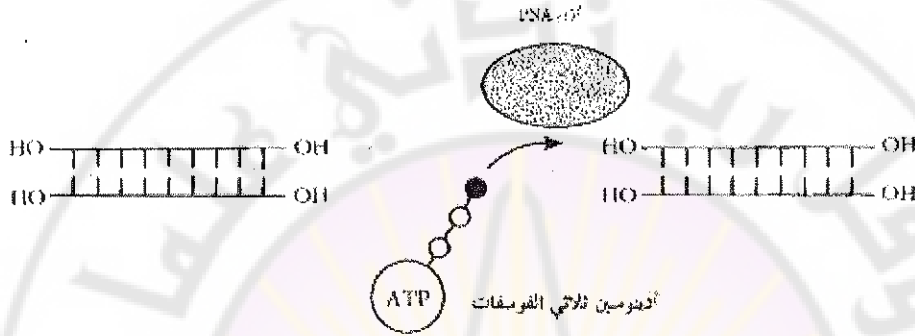
(شكل 41) يبين طريقة تشيع النهايات عن طريق استعمال أنزيم Polynucleotide kinase (PNK)
