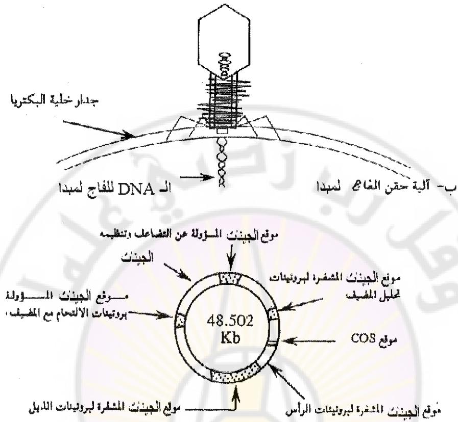
(شكل 61) يبين في الجزء العلوي الشكل العام للفاج لمبدأ طريقة العدوى، وفي الجزء السفلي الخريطة الوراثية لهذا الفاج
