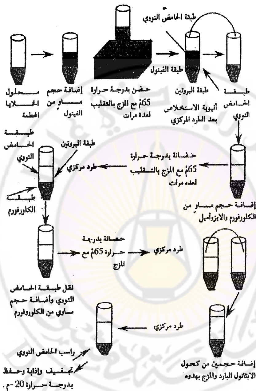
(شكل 40): يبين الطريقة التي يتم من خلالها عزل الـ DNA وتلقيته بشكل تفصيلي بواسطة الفينول والكلوروفورم والأيزوبرينول
