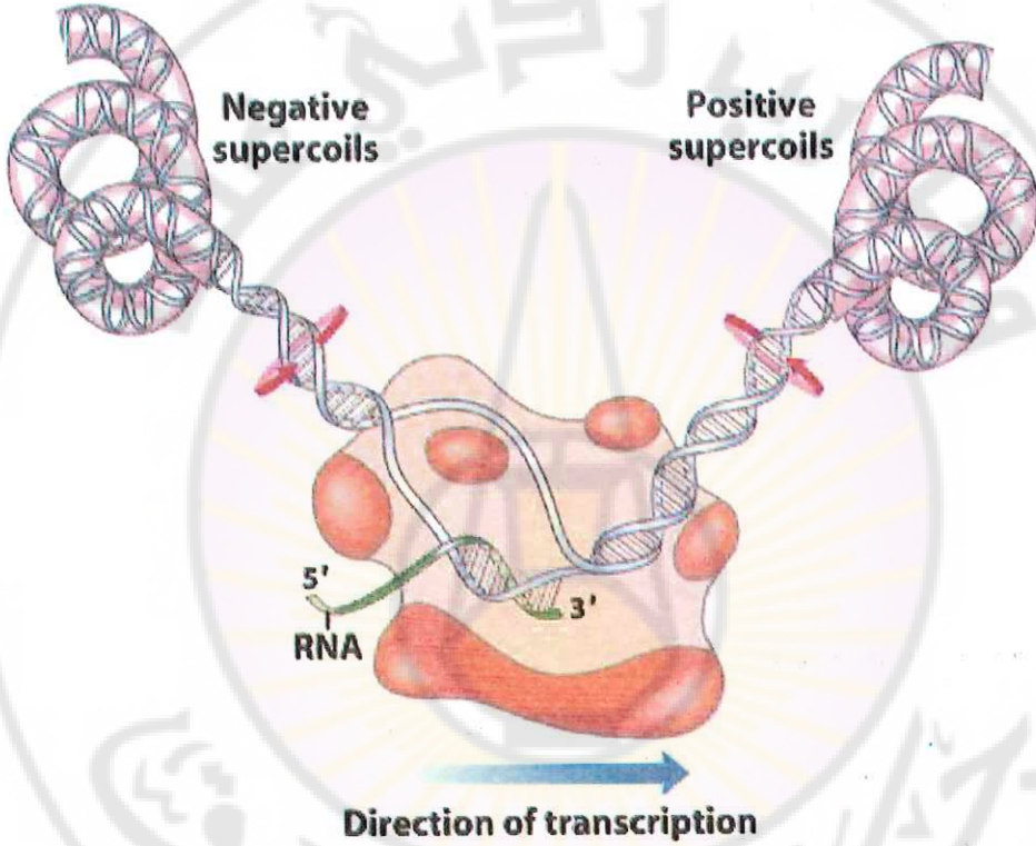
(شكل 23): يبين آلية نسخ الأنماط المختلفة من الـ RNA بدءاً من الـ DNA .
