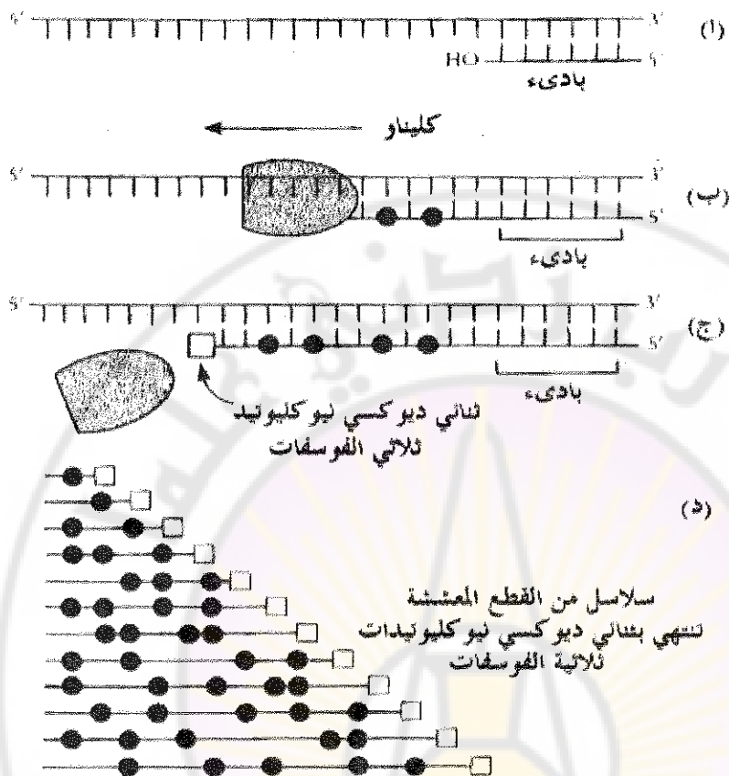
(شكل 49): يوضح طريقة سانجر وكولسون في الحصول على القطع المعشنة أنزيميا بهدف إنجاز عملية السلسلة لقطعة من الـ DNA.
