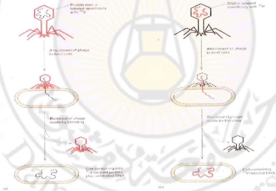
(شكل 3): يبين أن الطبيعة للمادة الوراثية في الفيروسات هي الـ DNA من خلال عملية الوسم لا DNA بواسطة الفوسفات المعلم للبروتين الغلافي بواسطة الكبريت المشع.
