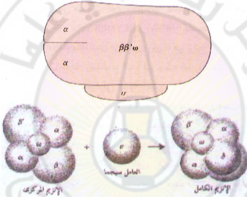
(شكل 22) يبين تخطيطاً لأنزيم RNA Polymerase والمؤلف من ست وحدات
