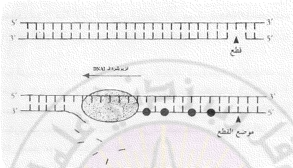
(شكل 42): يبين طريقة تشيع جزيء الـ DNA عن طريق الترجمة المتتمة باستعمال أنزيم كورنبرغ.
