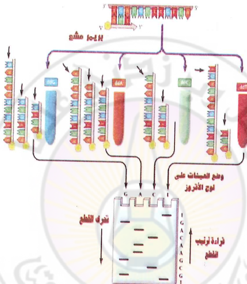
شكل (51-ب) يبين تفصيلاً لكيفية استعمال القطع المعشقة في الرحلان الكهربائي، ومن ثم قراءة السلسلة.
