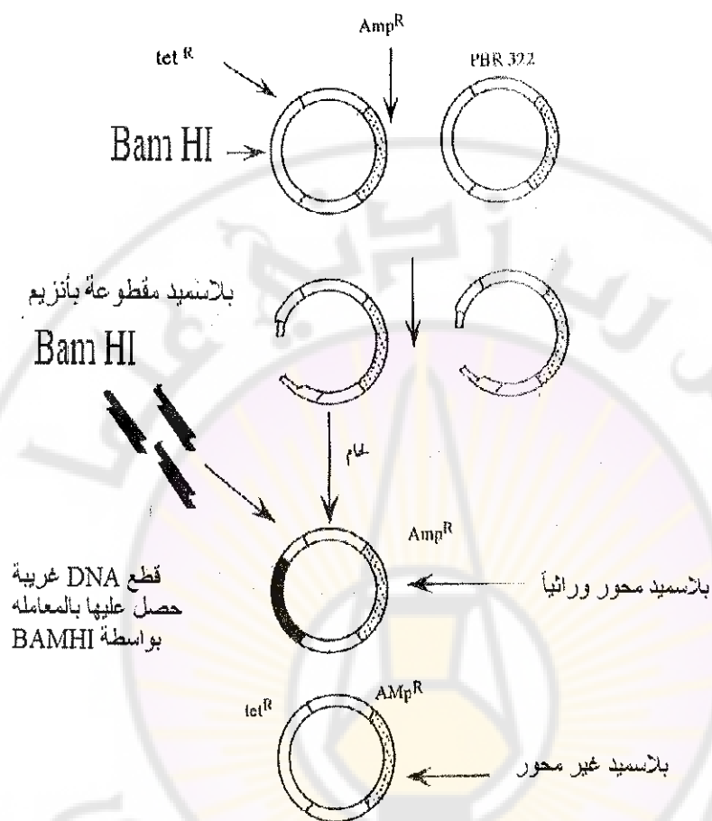
(شكل 53) يبين طريقة الغرس التثبيطي في جين التتراسكلين عند البلازميد .PBR322
