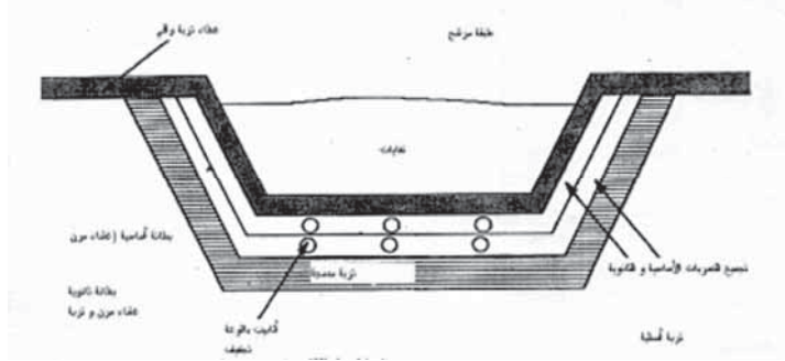
الشكل 2-24 قطاع عرضي في مكب نفايات آمن بنظام بطانة مزدوجة
