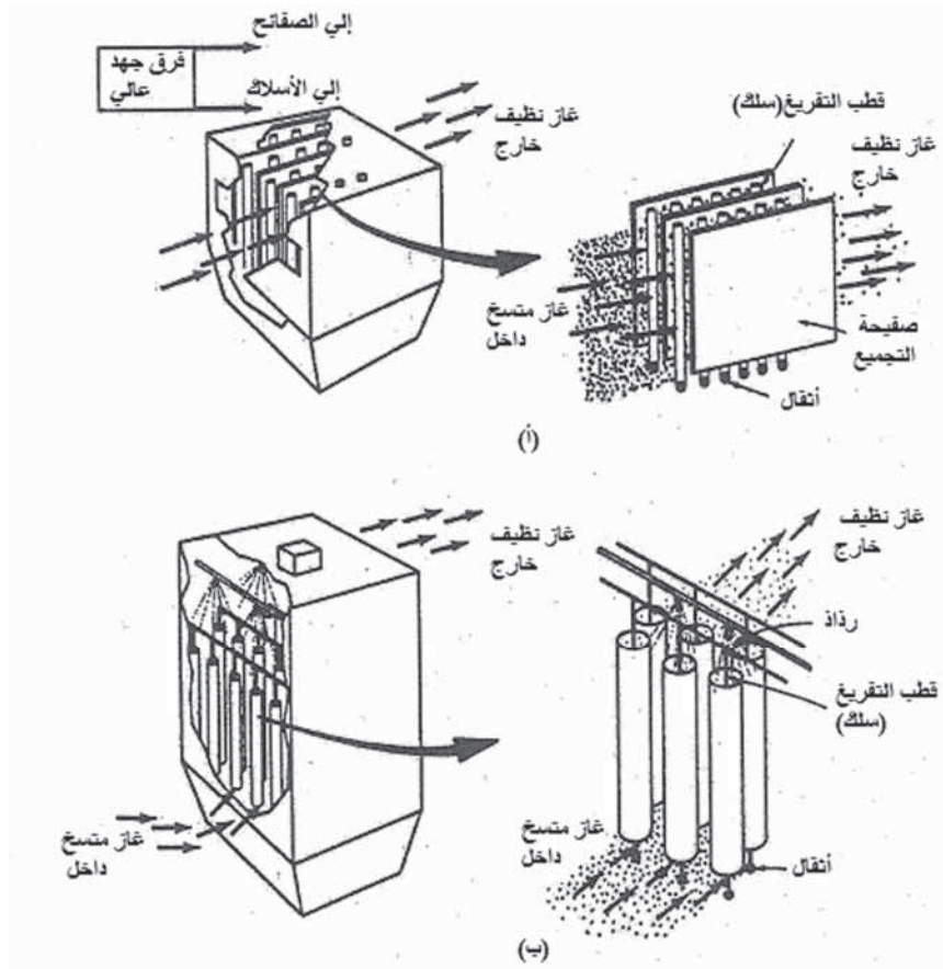
الشكل 5.14 المرسب الكهروستاتيكي (أ) النوع الطبقي و(ب) النوع الأنبوبي إي بي أي. تقنيات التحكم في الغازات والمواد الحبيبية، 1971
