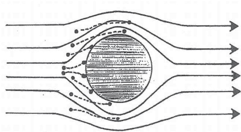
الشكل 1.14 تجمع الجسيمات على جسم ساكن
