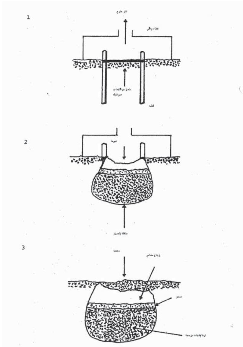
الشكل 21-7 تتابع عملية التزجيج الموضعية.
