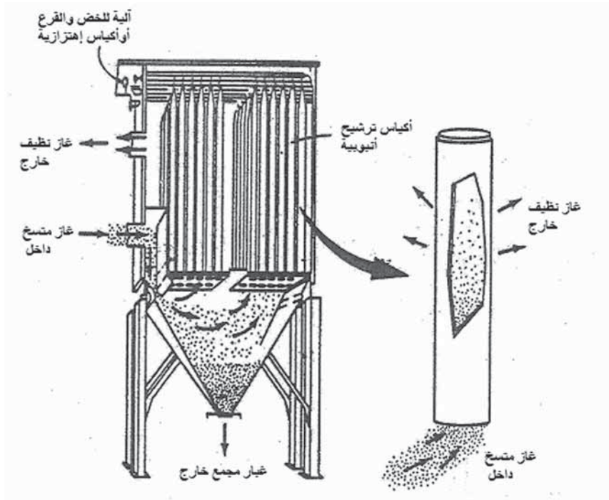
الشكل 7.14 نموذج لتصميم منقي قماشي بسيط إي بي أي. تقنيات التحكم في الغازات والمواد الحبيبية، 1971
