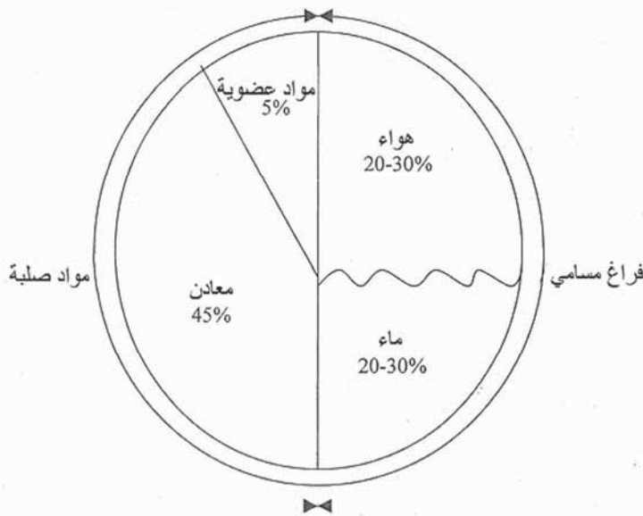
الشكل 1.6 التراكيز المعتادة في حجم من طبقة الطُفْل السطحية. يدل الخط المتموج بين الماء والهواء على أن النسب بين هذين المكونين تتذبذب كلما أصبحت التربة أكثر جفافاً أو أكثر رطوبة.
