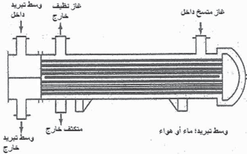
الشكل 11.14 مكثف سطحي اي بي أي تقنيات التحكم في الغازات والمواد الحبيبية، 1971.
