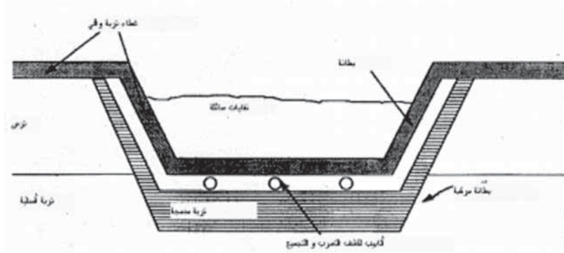
الشكل 1-24 قطاع عرضي لمحتجز سطحي لنفايات سائلة
