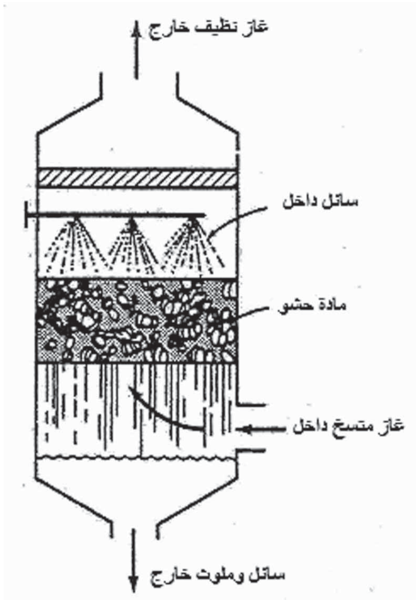
الشكل 8.14 نموذج لبرج معبأ به إنسياب للتيار للعكسي إي بي أي. تقنيات التحكم في الغازات والمواد الحبيبية، 1971
