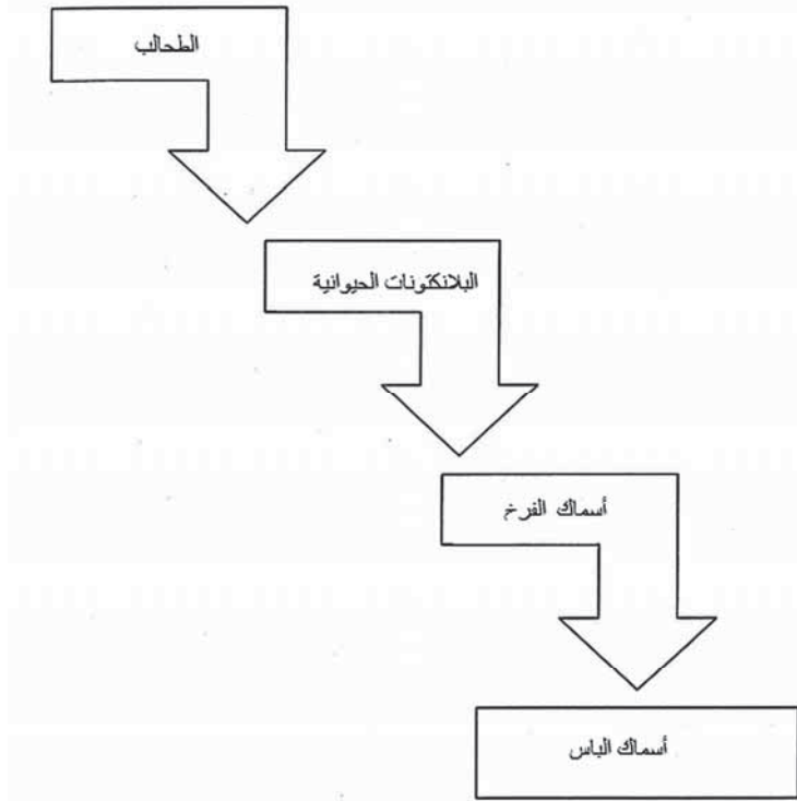
الشكل 7.2 سلسلة الغذاء المائية
