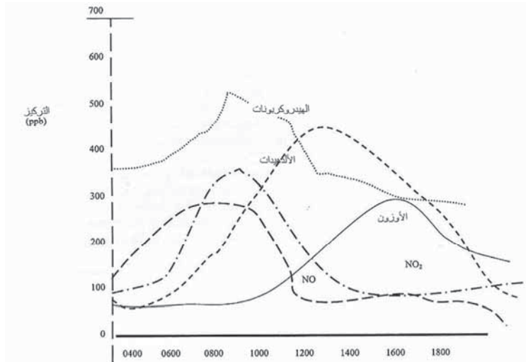
الشكل 3.11 متوسط التركيز لعدد من ملوثات الهواء في جو لوس أنجليس خلال الأيام التي يحدث فيها تهيج للعين.
