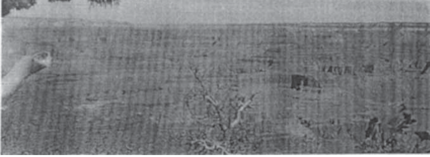
الشكل 7-16 ب. جراند كانيون
