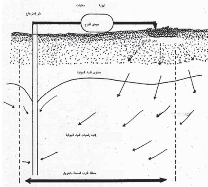
الشكل 5-21 مخطط التفكير الحيوي الموضعي - معبر الترشيح.
