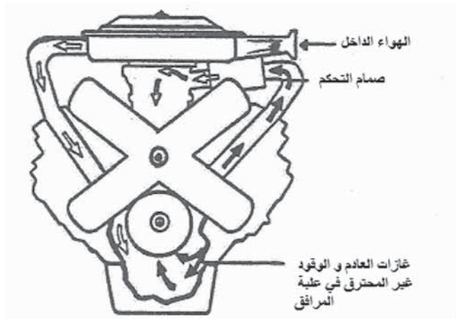
الشكل 19.14 تنفيس علبة المرافق الإيجابي لغازات الاحتراق المتسربة مأخوذ من: (T.Godish. Air Quality, 1997, p 290).
