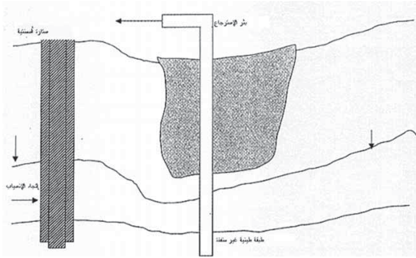
الشكل 9-21 ستارة أسمنتية.
