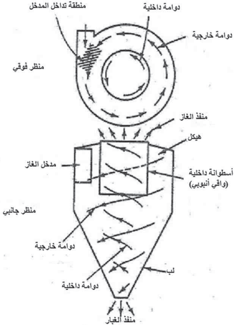
الشكل 4.14 زويدة الإنسياب المعكوس يو إس إتش إي دبليو. تقنيات التحكم في ملوثات الهواء الحبيبية
