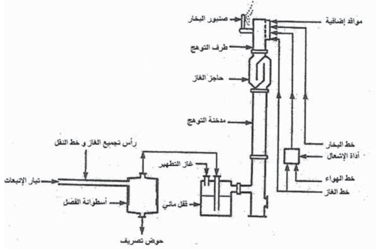
الشكل 14.14 مخطط توضيحي لنظام توهج مدعم بالبخار إي بي أي، دليل-تقنيات التحكم في ملوثات الهواء الخطرة، 1986.
