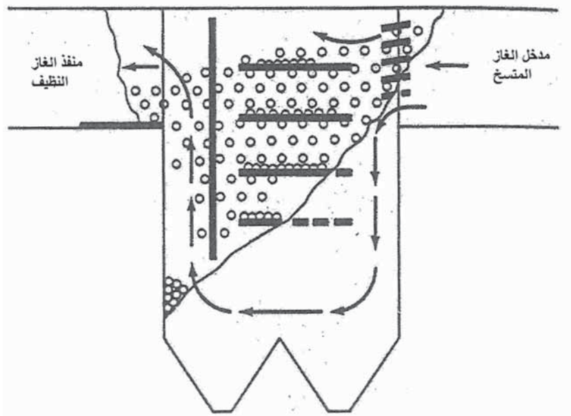
الشكل 3.14 غرفة ترسيب بفعل الجاذبية مكبوجة EPA تقنيات التحكم في الغازات والمواد الحبيبية، 1971
