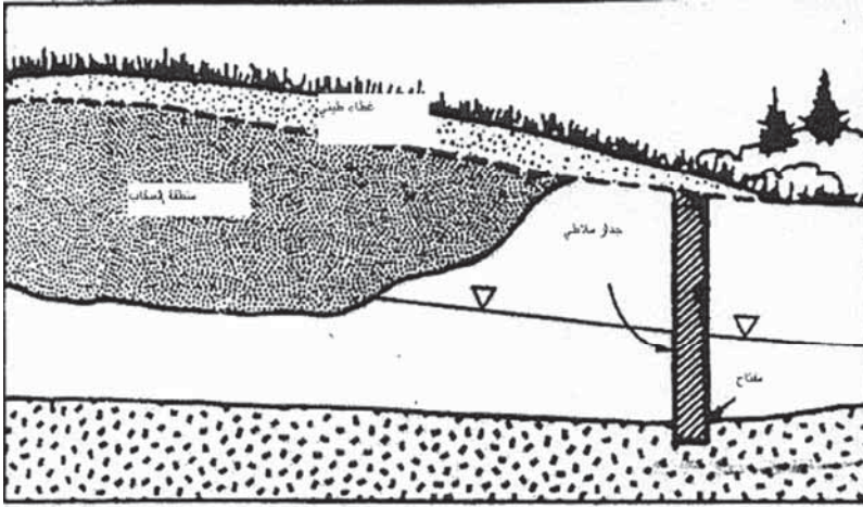
الشكل 8-21 جدار ملاطي معدل.
