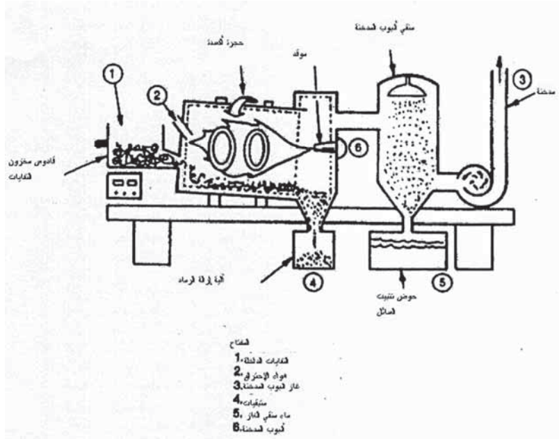
الشكل 21-11 مخطط موقد ترميد دوار
