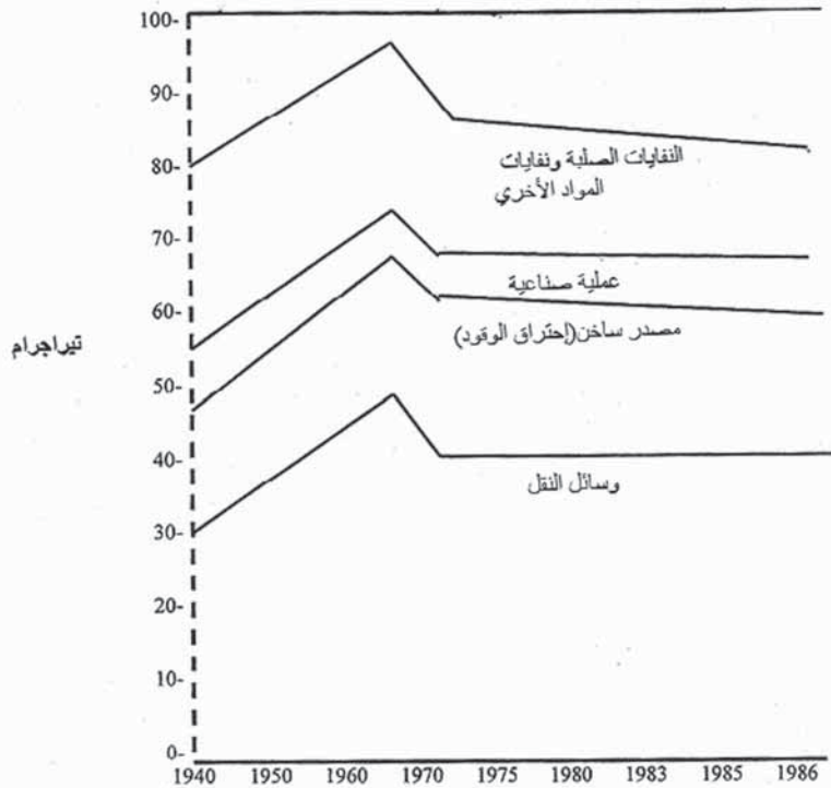
الشكل 2.11 نزعة إنبعاثات أول أكسيد الكربون، 1986-1940 مأخوذة من EPA التقديرات الوطنية لإنبعاثات ملوثات الهواء 1986-1940، 1988.
