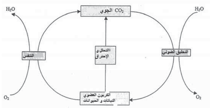
الشكل 1.2 دورة الكربون
