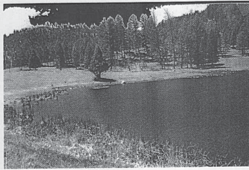
الشكل 16-8 منطقة البركة في نهر بمنطقة أكستر، جنوب داكوتا
