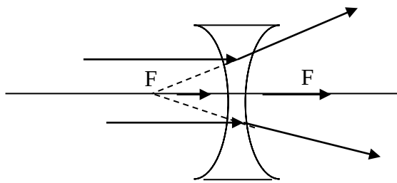
شكل (١٠-٥-٢) عدسة مقعرة أو مفرقة
