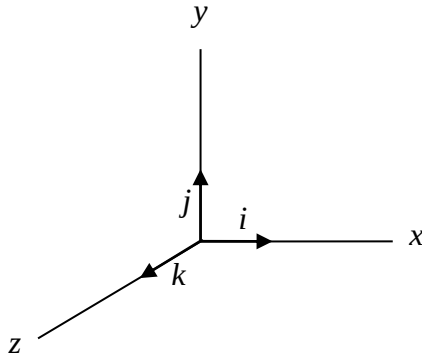
شكل (١٠-٢) متجهات الوحدة \mathbf{i} و \mathbf{j} و \mathbf{k} تتجه في الاتجاه الموجب للمحاور الثلاثة x و y و z على الترتيب
