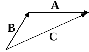
شكل (٦-٢) محصلة متجهين B+A بطريقة المثلث
