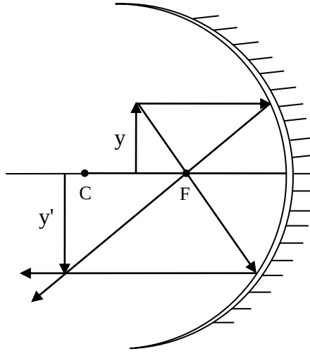
شكل (٣-٨-٥) عندما يكون الجسم بين مركز التكور والبؤرة تتكون صورة حقيقية مقلوبة اكبر من طول الجسم
