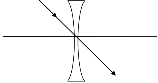
شكل (٥-١٢-١) الشعاع الذي يسقط مارا بمركز العدسة لا يعاني أي انكسار
