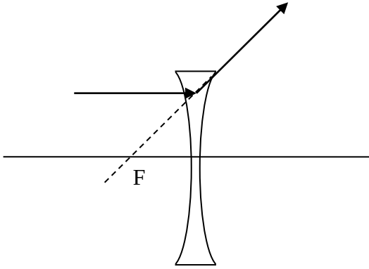
شكل (٥-١٢-٢) الشعاع الذي يسقط موازيا للمحور الأصلي للعدسة ينكسر بحيث يمر امتداده بالبؤرة
