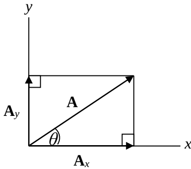
شكل (١١-٢) تحليل المتجه \mathbf{A} إلى مركبتين متعامدتين
