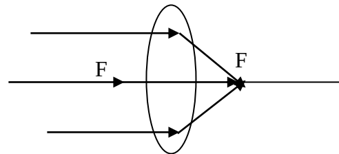
شكل (١٠-٥-١) عدسة محدبة أو لامة
