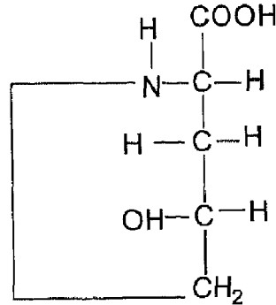
L-OH Proline
