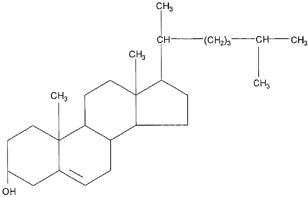
Cholesterol (كولسترول)
