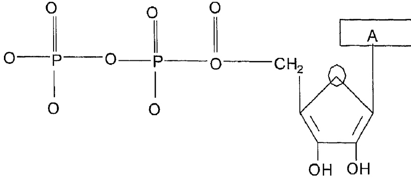
ATP
