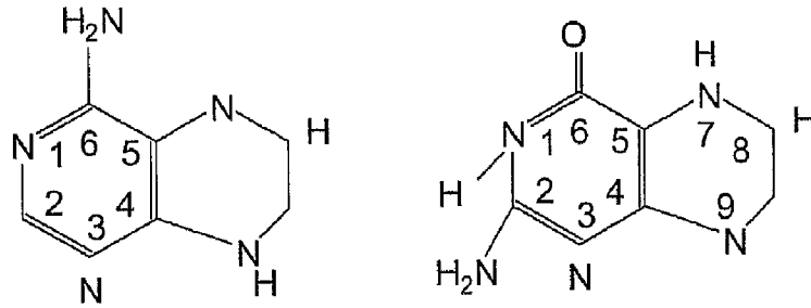
(A)Adenine)
