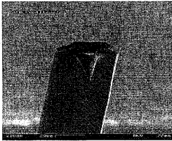
شكل (42) صورة توضح ذراع AFM ويبلغ عرضه 100 ميكرومتر ويمكن ان يصل إلى 20 ميكرومتر او أقل.
