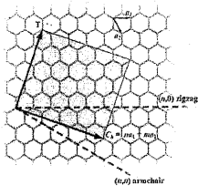
شكل (22) أنواع الأنابيب النانوية الكربونية الاحادية وميكلها البنائية
