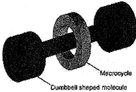
شكل (16) توضيحي للروتاكسان، المستخدم كمقلاد (مبدال) جزيئي.
