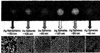
شكل (1) تغير لون محلول جسيمات النانو الذهبية وكذلك محلول جسيمات النانو الفضية وذلك تبعا لتغير احجام واشكال هذه الجسيمات
