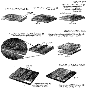
شكل (37) الليثوغرافيا اللينة
