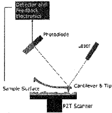
شكل (41) مخطط توضيحي لفكرة عمل ميكروسكوب القوة الذرية
