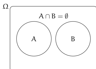
FIGURA 9.5: Due eventi A e B si dicono incompatibili , se il verificarsi dell'uno esclude il verificarsi dell'altro.
