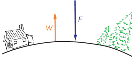
الشكل 4-5 بيان القوى المؤثرة على الأرض.
