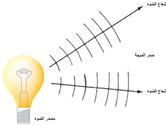
الشكل ج-1 أشعة الضوء تكون عمودية على صدر الموجة.
