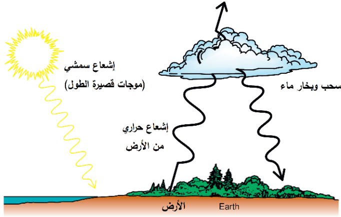
الشكل 18-1: تأثير البيت الزجاجي (الدفيئة أو الاحتباس الحراري).
