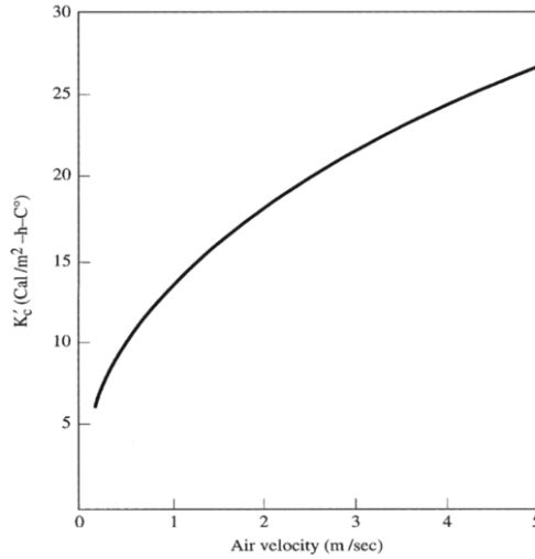
الشكل 16-1: معامل الحمل الحراري كدالة في سرعة الهواء.
