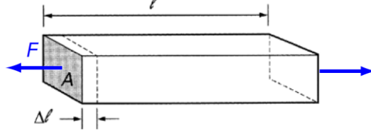
الشكل 5-1 استطالة قضيب نتيجة قوة مطبقة.
