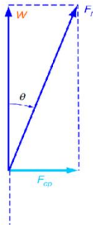
الشكل 8-4: منعطف مائل.
