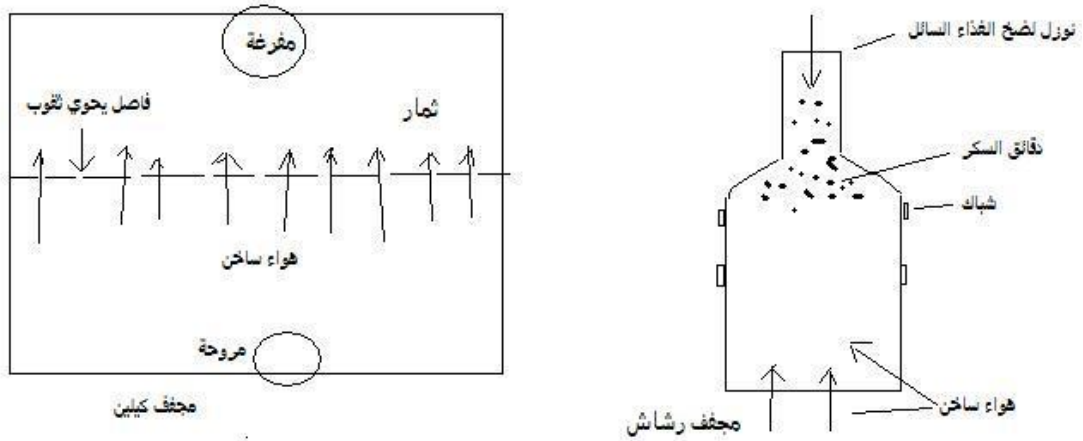
شكل (68) مجففات كيلين
