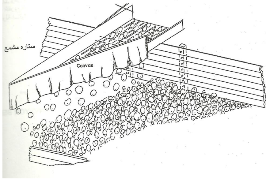
شكل (14) فرز المحاصيل البستانية باستخدام الماء .
