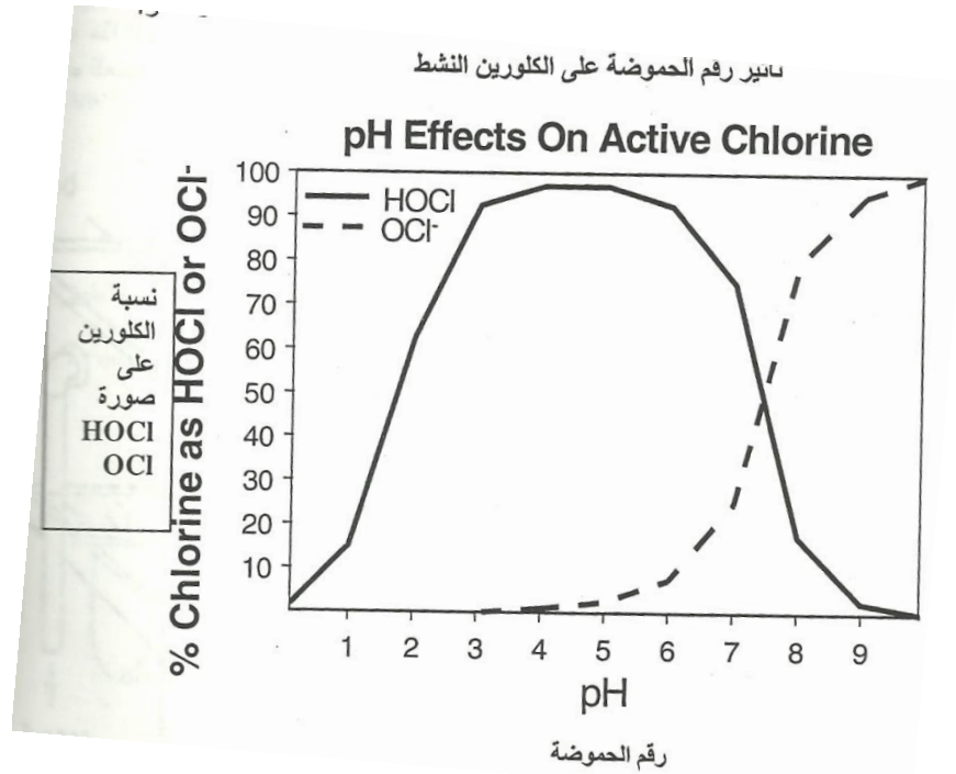
شكل (19) العلاقة بين PH وفعالية الكلورين
