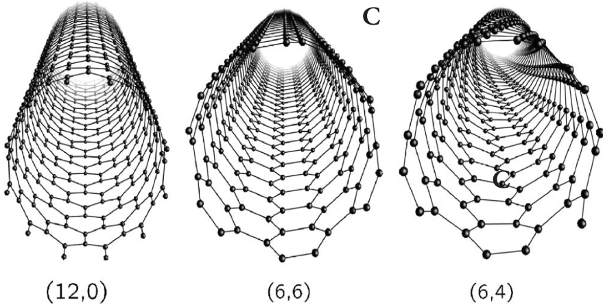
شكل رقم (٣-٢٤) Zigzag (يسار)، Armchair (وسط)، Chiral (يمين) (٤٥).
