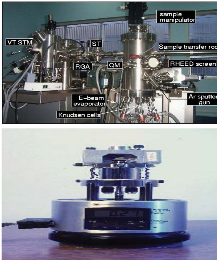
شكل رقم (٢-٢٣) المجهر النفقي الماسح (STM) (٢٤).
