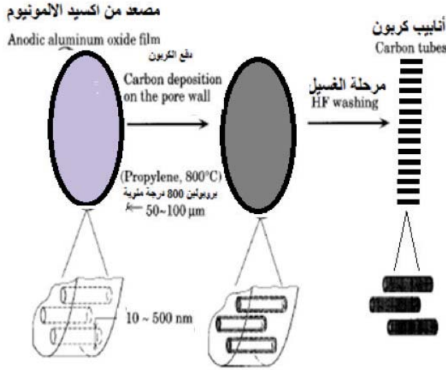
شكل رقم (٣-١٦) مخطط توضيحي لعمليات تصنيع أنابيب الكربون النانوية باستخدام طريقة الترسيب البخاري في مسامات أكسيد الألومنيوم (٢٤).
