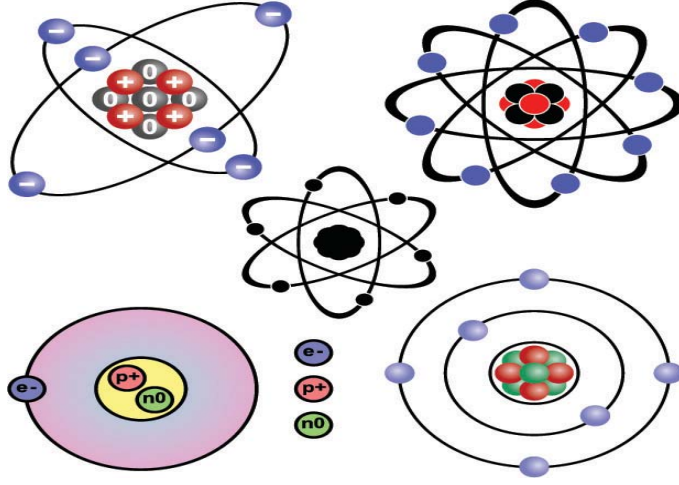
شكل رقم (١-٢) الإلكترونات حول النواة لذرة الكربون (٩٢).
