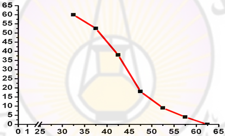
الشكل (8-7): المنحني التكراري المتجمع النازل
