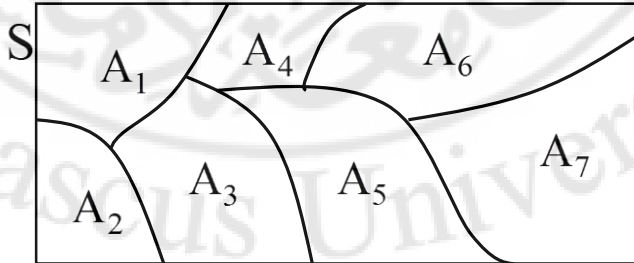
الشكل (22-8) يوضح تجزئة لفضاء التجربة S
