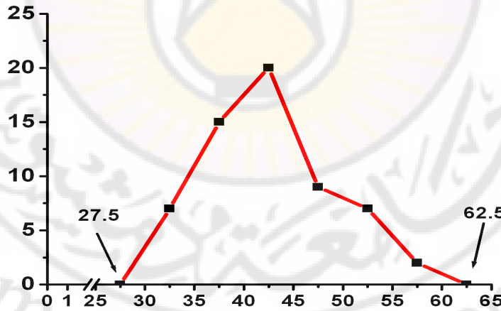
الشكل (5-8): المنحني التكراري
