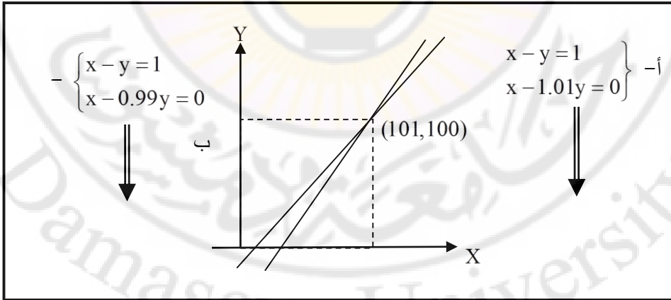
الشكل (9-3) المستقيمان متوازنان تقريباً
