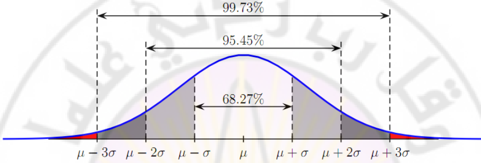
الشكل (8-20): توضيح للقاعدة التجريبية
