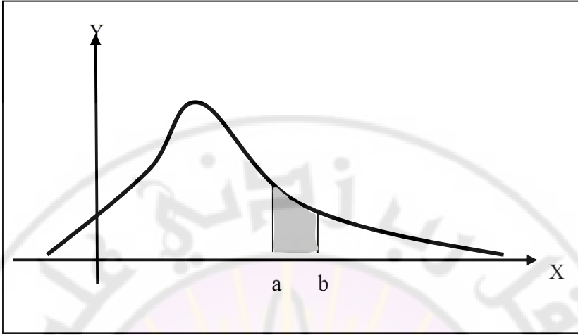
الشكل (8-25) - مساحة المنطقة المظلمة تمثل الاحتمال P(a \leq X \leq b)
