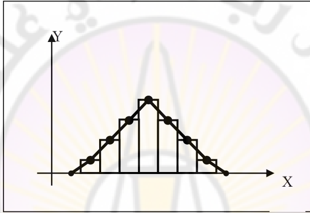
الشكل (8-12): توزيع تكراري متماثل أو معتدل فيه \bar{x} = M = \tilde{x} ودرجة الالتواء صفر
