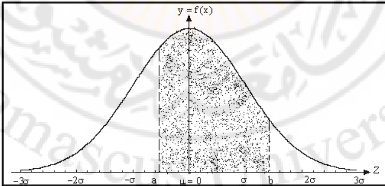
الشكل (8-32): المنحني الطبيعي المعياري الذي يمثل التوزيع الطبيعي المعياري N(0,1)
