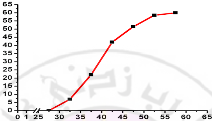
الشكل (8-6): المنحني التكراري المتجمع الصاعد
