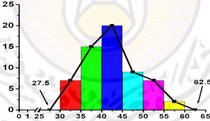
الشكل (8.1): المدرج التكراري والمضلع التكراري (الخط المنكسر)
