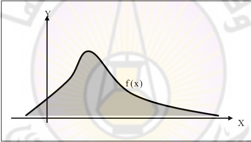
الشكل (8-24) - مساحة المنطقة المظللة = 1
