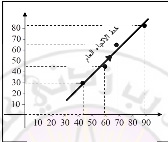
الشكل (8.40) - الشكل الانتشاري للمثال (52)
