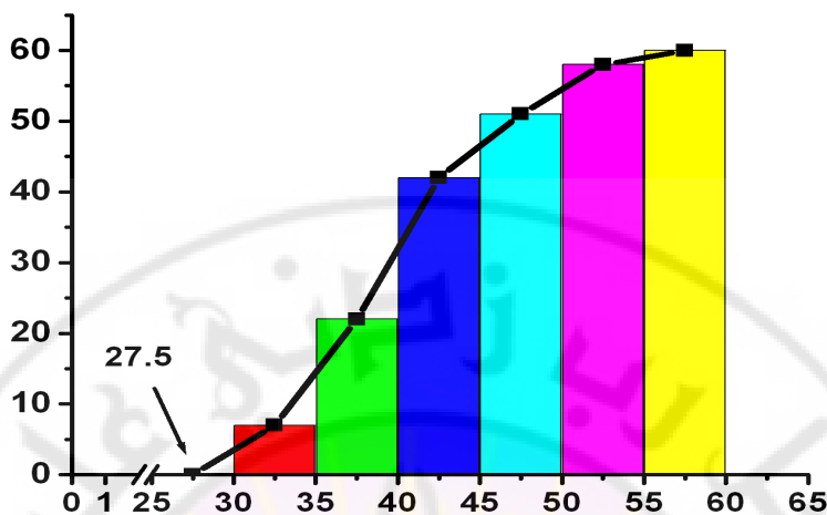
الشكل (3-8): المدرج (المضلع) التكراري المتجمع الصاعد
