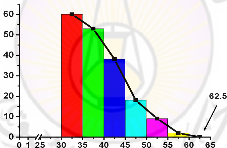
الشكل (4-8): المدرج (المضلع) التكراري المتجمع النازل
