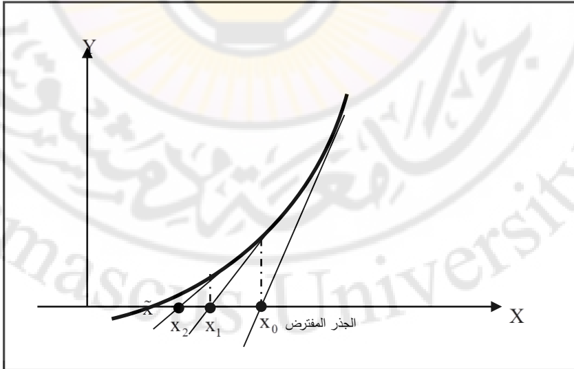
الشكل (2-9) يوضح النقاط القاطعة للمحور X التي تمثل متتالية الحلول التقريبية.
